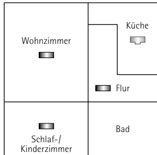
Abb. 2 ■ Rauchwarnmelder ■ Wärmewarnmelder
